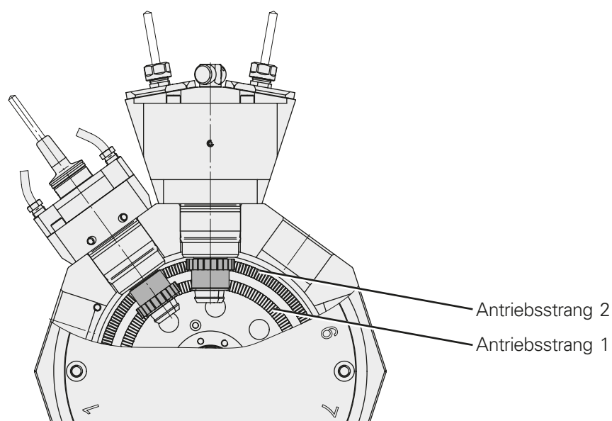
Werkzeugrevolver oben und unten
