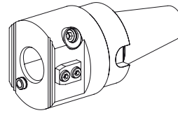
Voreinstelladapter Steilkegel 50
