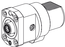
Voreinstelladapter VDI80 Werkzeugaufnahme HSK63 Artikel-Nr. 10094249
