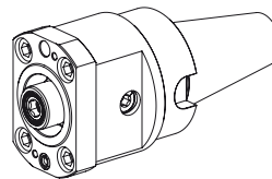
Voreinstelladapter Steilkegel 50 Werkzeugaufnahme HSK63 Artikel-Nr. 10614276
