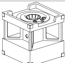
Voreinstellklotz Grundkörper Artikel-Nr. 10444808
