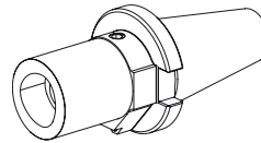
Voreinstelladapter Steilkegel 50 Werkzeugaufnahme CAPTO C6 Artikel-Nr. 12095573
