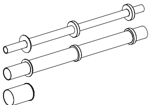
Spindeldurchlass 120mm Spannhub 48mm Materialdurchmesser D40 - D120
