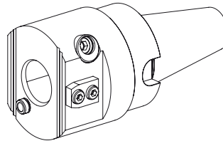
Voreinstelladapter Steilkegel 50
