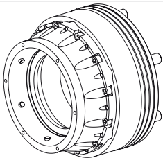
Hainbuch Spanntop nova Futter, Modular
