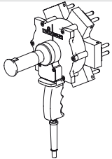
Hainbuch, Wechsellvorrichtung pneumatisch Spanntop nova Futter
