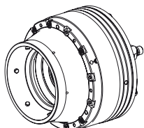
Hainbuch Spanntop mini Futter, Kombi Axzug
