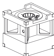
Voreinstellklotz
