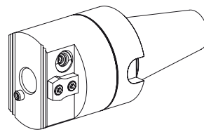
Voreinstelladapter Steilkegel 50
