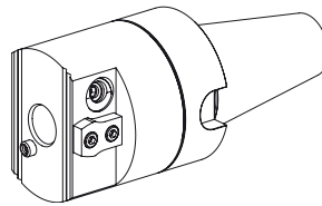
Voreinstelladapter Steilkegel 50 Werkzeugaufnahme VDI25 Artikel-Nr. 10622335
