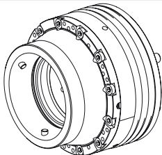
Hainbuch Spanntop mini chuck, Kombi Axfix
