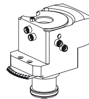
Cube de pré-réglage
