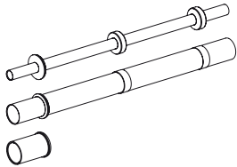
Diamètre de broche 65mm, Course serrage sans objet
