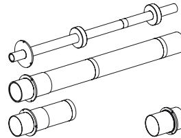
Diamètre de broche 90mm, Course serrage 10mm
