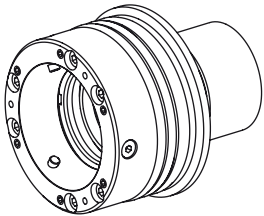
Broche principale D65 Hainbuch Spanntop nova mandrin, Modulaire
