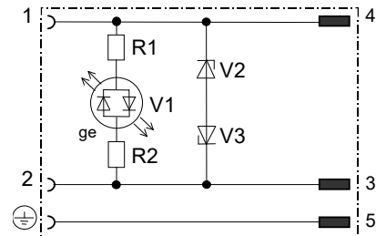
STROMLAUFPLAN Schematic diagram
