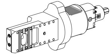
Adapter für Voreinstellgeräte
