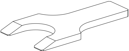
Abziehvorrichtung
