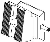
Schwalbenschwanzaufnahme (ABC)
