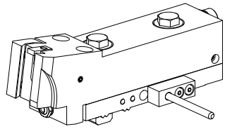
MS16 grooving slide
