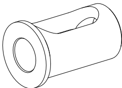
Douille attachement collerette
