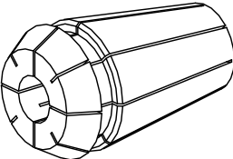
ER-Gewindebohrspannzange
