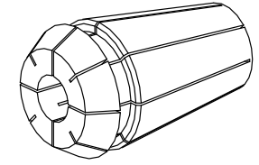
ER-Gewindebohrspannzange
