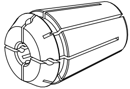
ER-Spannzange, abgedichtet
