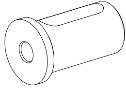
Aufnahmebuchse mit Bund
