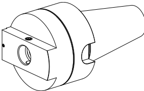
Adapter für Voreinstellgeräte
