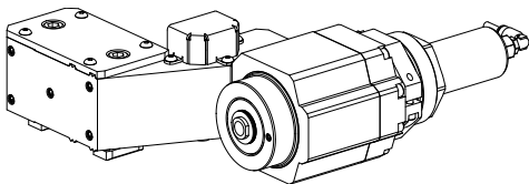
MS16 grooving slide
