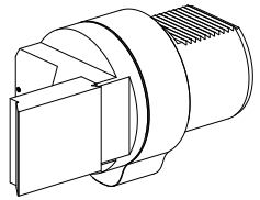
Adapter für Voreinstellgeräte
